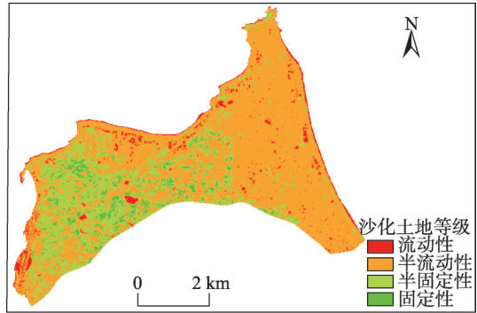
注: 流动性、半流动性、半固定性、固定性土地的沙化等级依次是4、3、2、1。
