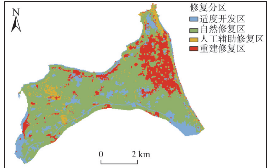
图9 木兰湾沙化灾害生态修复分区
