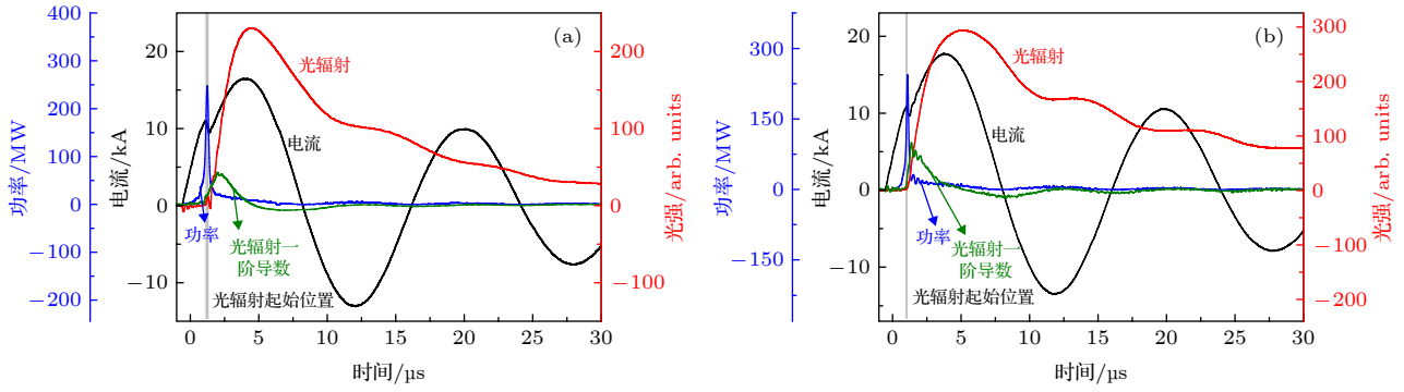
图5 铜单丝与丝阵负载电流、功率、光辐、及光辐射一阶导数波形图 (a) 铜单丝 200 μm; (b) 铜丝阵 4 根
