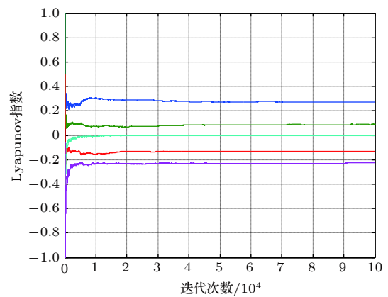
图 1 Lyapunov 指数谱
