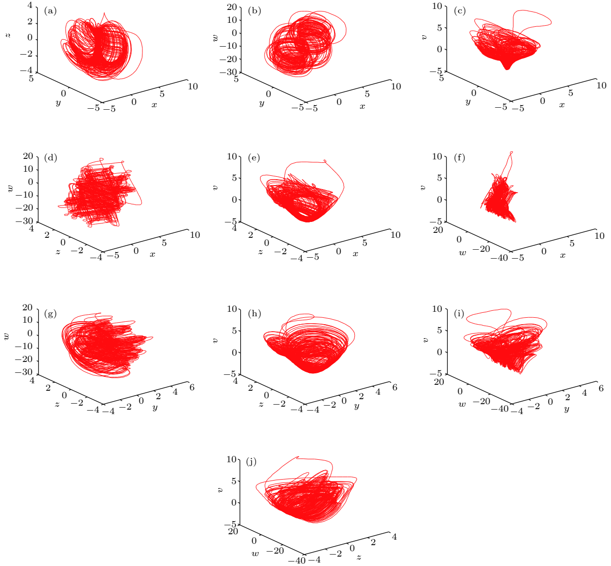
图 4 三维相图 (a) x-y-z 三维图; (b) x-y-w 三维图; (c) x-y-v 三维图; (d) x-z-w 三维图; (e) x-z-v 三维图; (f) x-w-v 三维图; (g) y-z-w 三维图; (h) y-z-v 三维图; (i) y-w-v 三维图; (j) z-w-v 三维图
