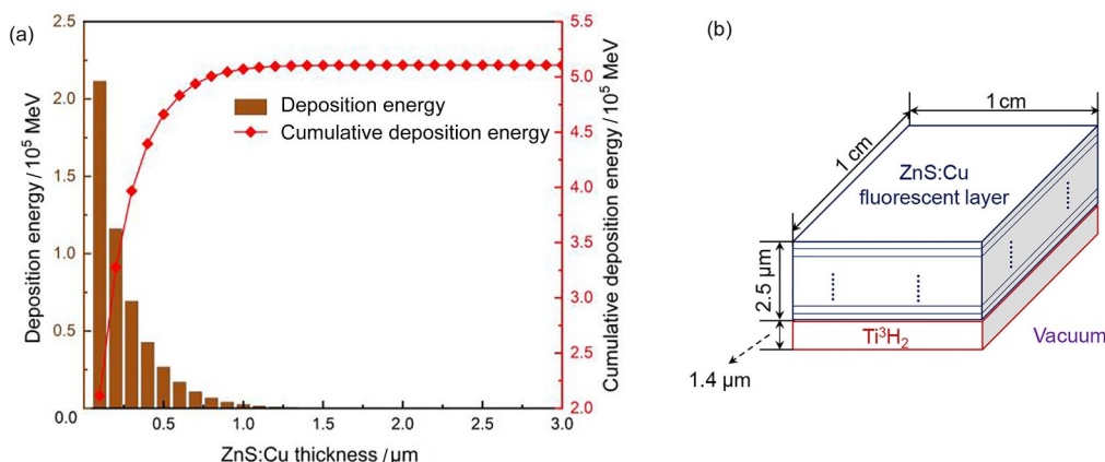
图 6 ZnS : Cu 荧光层中沉积能量分布和累计沉积能量随材料厚度的变化趋势 (a) 与 ZnS : Cu 荧光层辐致发光计算模型 (b) Fig. 6 Distribution of deposition energy and cumulative deposition energy (a), and radioluminescence calculation model in ZnS : Cu fluorescent layer (b)
