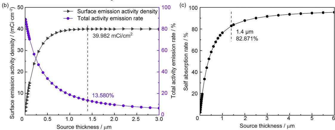
图 2 Ti^3H_2 源的表面出射功率密度、总功率出射率(a)；表面出射活度密度、总活度出射率(b)；自吸收率随源厚度的变化趋势(c)
