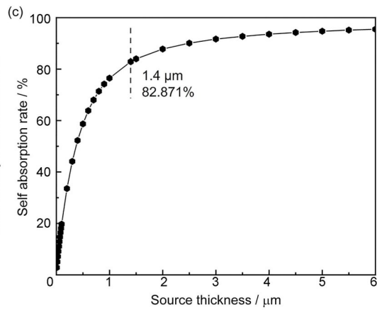
图 2 Ti^3H_2 源的表面出射功率密度、总功率出射率(a)；表面出射活度密度、总活度出射率(b)；自吸收率随源厚度的变化趋势(c)
