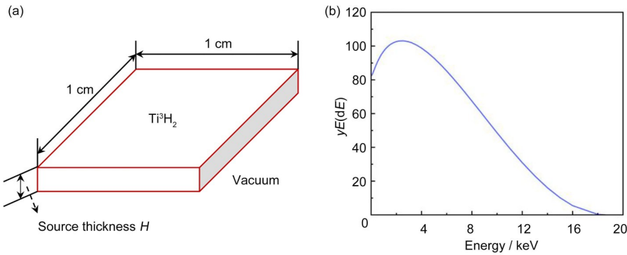
图 1 (a) Ti^3H_2 同位素源模型；(b) ^3H 的微分能谱
