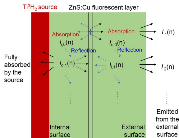
图 7 ZnS : Cu 荧光层中荧光的运输过程 Fig. 7 Fluorescence transport process in ZnS : Cu fluorescent layer
