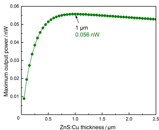
图9 基于 Si 半导体光伏组件和 \text{Ti}^3\text{H}_2 源的辐致光伏效应氚基同位素电池的最大输出功率随荧光层厚度的变化趋势
