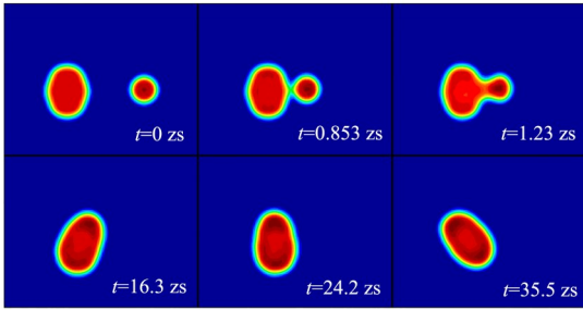
图5 TDHF 模型计算融合反应 ^{50}\text{Ti}+^{249}\text{Bk} 的质量密度随时间演化图像 [44]
