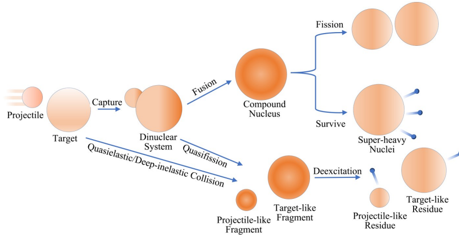
图2 基于DNS模型描述的融合反应和多核子转移反应不同阶段示意图 Fig.2 Schematic illustration of fusion and MNT reactions within the DNS model framework
