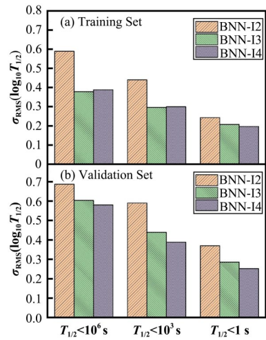
图1 训练集(a)和验证集(b)中三种神经网络BNN-I2、BNN-I3和BNN-I4计算的 \beta 衰变寿命与实验值的均方根偏差 \sigma_{\text{RMS}}(\lg T_{1/2})
