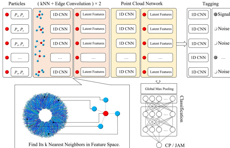
图7 使用动态棱卷积网络寻找动量空间的临界自相似信号,并标注存在临界关联的粒子 [39]
