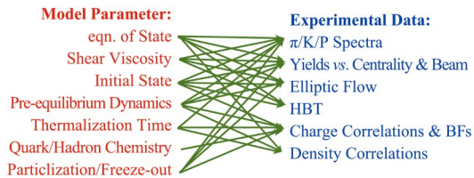
图1 通过高能核碰撞实验与理论模型对比提取核物质状态方程所遭遇的困难 [4]
