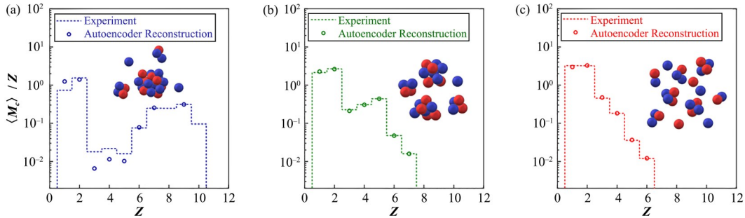
图 10 使用自编码器从重离子碰撞实验数据中学习,进行核液气分类 [46]
