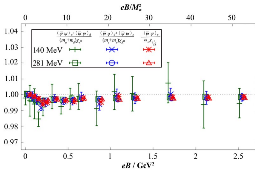
图9 Ward-Takahashi恒等式在温度为140 MeV和218 MeV的格点QCD的数值验证 [33]
