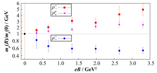
图2 自旋平行于磁场带正电的 \rho 介子, 自旋反平行于磁场的带正电的 \rho 介子以及中性的 \rho 介子与它们各自在磁场为零时的质量之比随磁场强度 eB 的变化 [24] 这些连续外推的结果基于淬火近似下的QCD组态, 采用的价夸克对应的pion的质量为415 MeV
