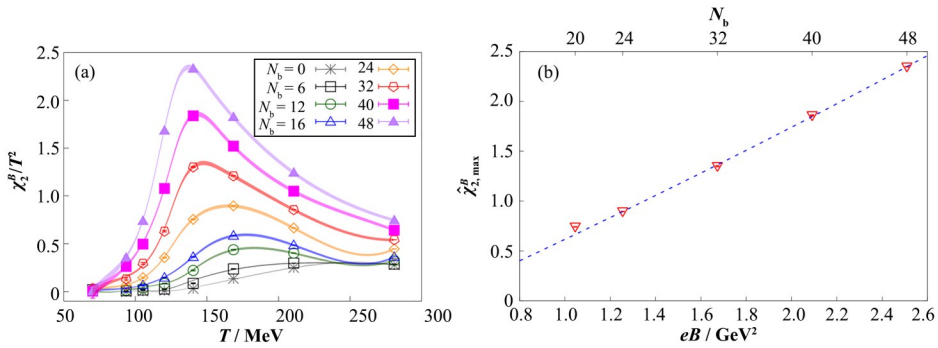
图13 二阶重子数涨落在不同磁场强度下随温度的变化关系(a) [52] ,根据二阶重子数涨落的临界行为拟合峰的高度得到临界点处磁场强度约为 7 \text{ GeV}^2 (b)
