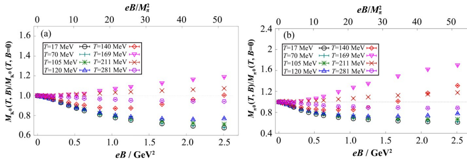
图10 中性膺标量介子的屏蔽质量在磁场不为零时的结果与磁场为零时的结果的比值在不同温度随磁场强度的变化 [33] (a) 中性pion的结果, (b) 中性kaon的结果
