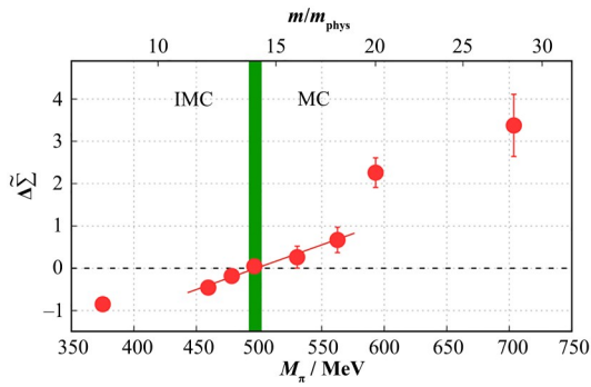
图7 手征凝聚在磁场为 0.6 \text{ GeV}^2 时候与零磁场时的差别随 pion 介子质量的变化关系,温度取为随 pion 介子质量变化的赝临界温度值 [34]
