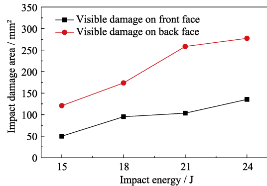
图 6 不同能量冲击后材料的损伤面积
