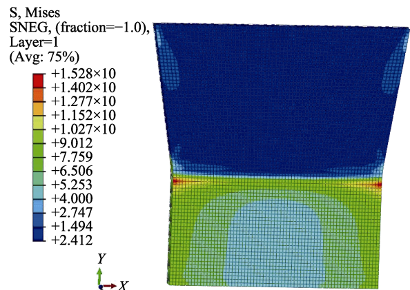
图 2 试样应力分布云图
