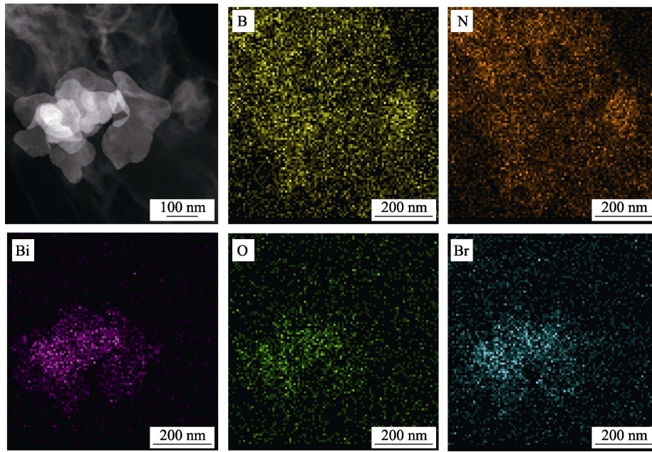
图 S6 5%BiOBr-BN 的 TEM-EDS 元素分布图 Fig. S6 TEM-EDS element mappings of the as-prepared 5%BiOBr-BN
