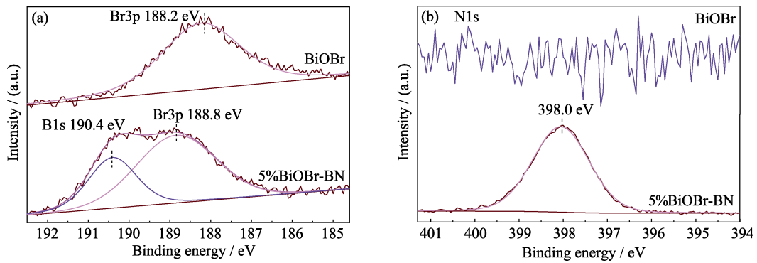
图 S7 BiOBr 及 5%BiOBr-BN 样品 XPS 图谱 Fig. S7 XPS spectra of the BiOBr and 5%BiOBr-BN composite
