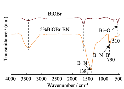
图 4 BiOBr 和 5%BiOBr-BN 的红外谱图 Fig. 4 FT-IR spectra of BiOBr and 5%BiOBr-BN
