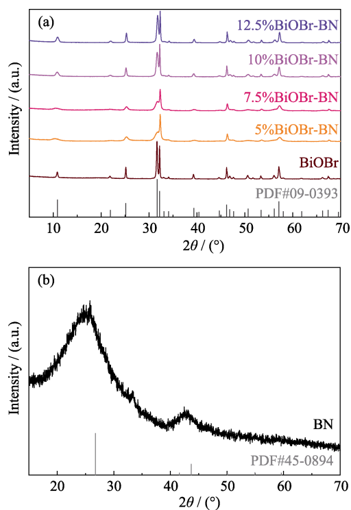
图 2 BiOBr, BiOBr-BN(a) 和 BN(b) 的 XRD 图谱 Fig. 2 XRD patterns of pure BiOBr, BiOBr-BN composites (a), and pure BN (b)
