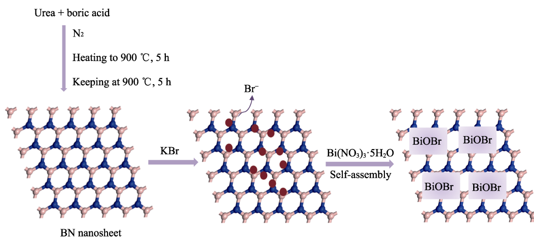
图 S1 BiOBr-BN 样品的形成过程示意图
