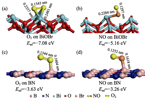
图 9 (a)O 2 和(b)NO 在 BiOBr 表面吸附构型; (c)O 2 和(d)NO 在 BN 表面吸附构型 Fig. 9 Optimized structure of (a) O 2 and (b) NO on BiOBr; optimized structure of (c) O 2 and (d) NO adsorbed on BN
