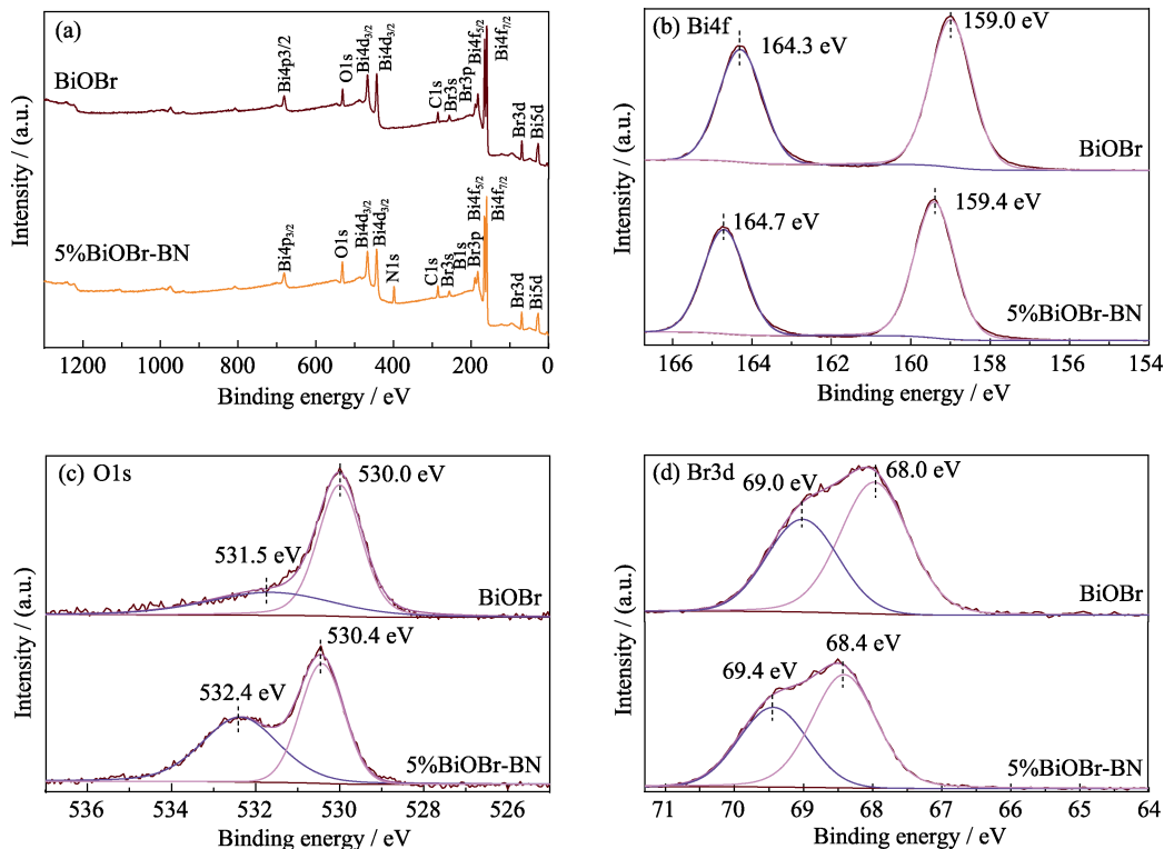
图 5 BiOBr 及 5%BiOBr-BN 样品 XPS 图谱 Fig. 5 XPS spectra of BiOBr and 5% BiOBr-BN composite
