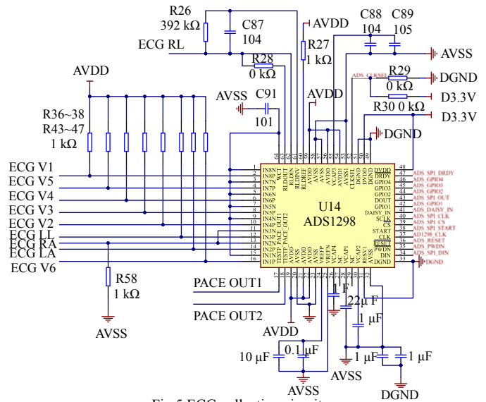
Fig.5 ECG collection circuit 图 5 心电采集电路
