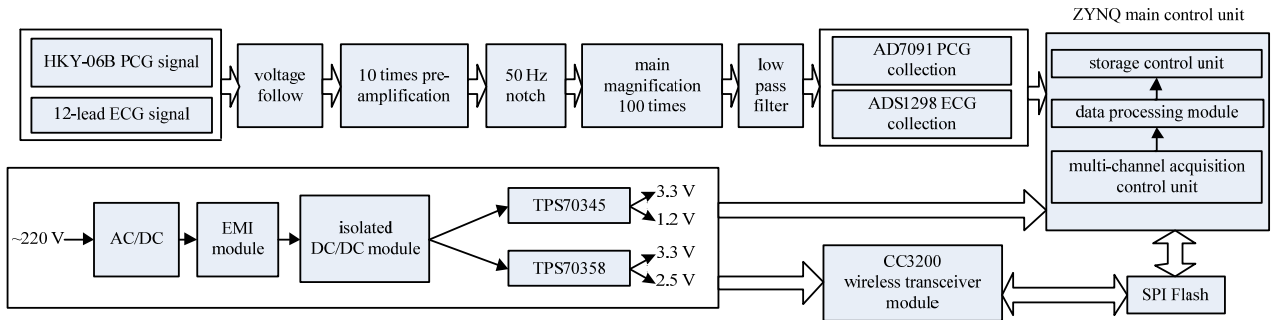
Fig.2 Structure diagram of a single node 图 2 单个节点组成结构框图
