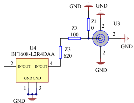
Fig.6 Radio frequency circuit 图 6 无线射频电路
