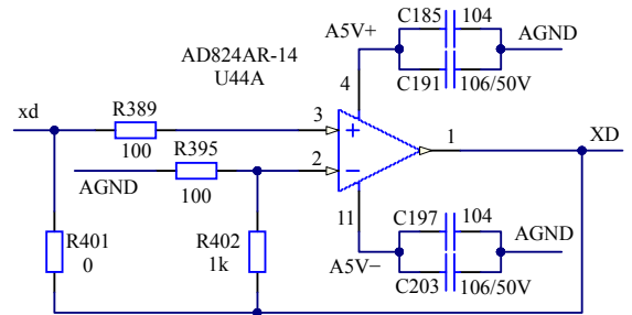
Fig.3 AD824 preamplifier circuit 图 3 AD824 前置放大电路
