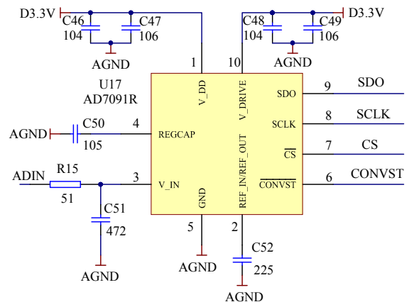
Fig.4 PCG collection circuit 图 4 心音采集电路
