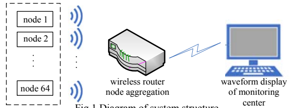
Fig.1 Diagram of system structure 图 1 系统组成结构示意图
