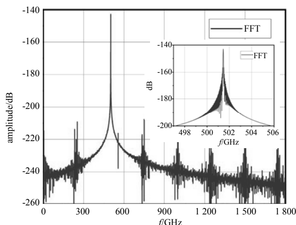
Fig.12 FFT spectrum of the output power 图 12 输出功率频谱图
