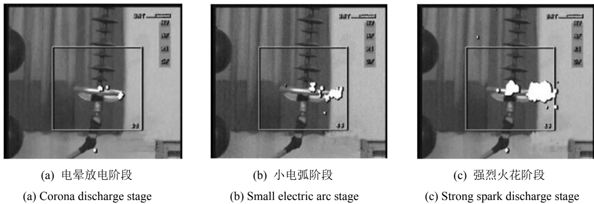
图5 均压环电晕放电紫外图像
