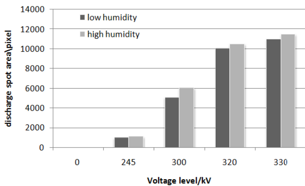
图6 不同湿度情况下光斑面积变化
