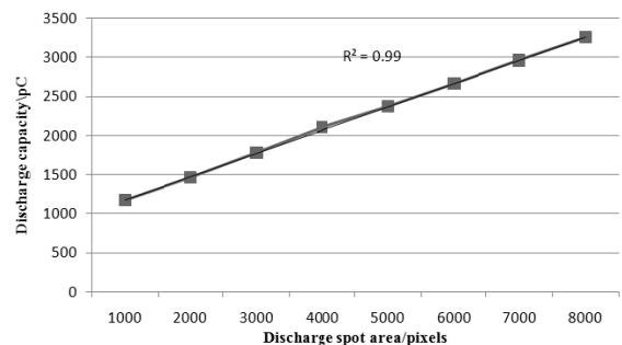
图 4 光斑面积与放电容量的关系曲线
