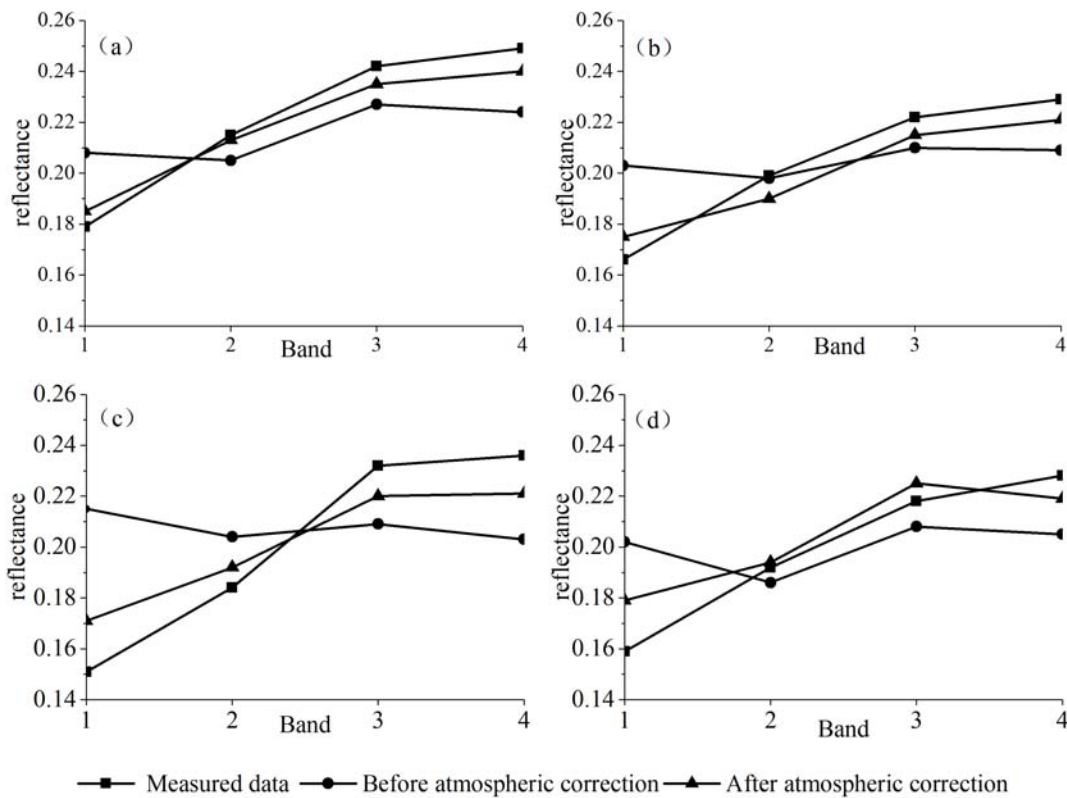
图6 高分二号影像大气校正前后反射率比较：图(a)~(d)分别代表 S1~S4 四个点反射率
