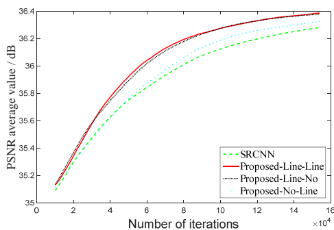
图5 2倍率下不同添加方式的线性灰度变换 PSNR 曲线
