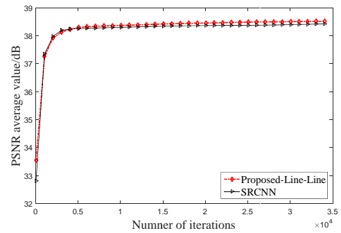
图 7 3 倍率下不同算法的 PSNR 曲线
