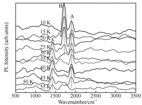
图 2 用 MBE 方法生长的 InSb 外延材料的变温 PL 光谱。其中, 垂直方向上的虚线表示不同能级间跃迁随温度的变化
