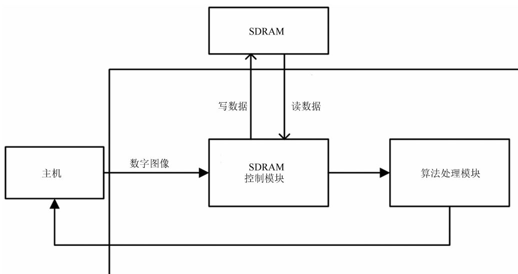
图4 系统结构图
