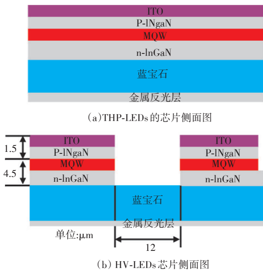
图1 THP-LEDs 的芯片侧面图和 HV-LEDs 芯片侧面图
