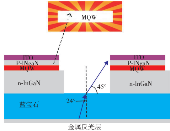
图8 HV-LEDs芯片间隙出光示意图
