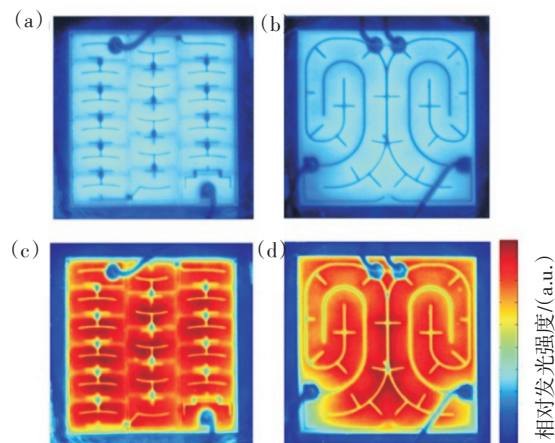
图6 (a) HV-LEDs和(b) THP-LEDs在1 W输入功率下的芯片发光强度图 (c) HV-LEDs和(d) THP-LEDs经过MATLAB图像处理后的芯片灰度图
