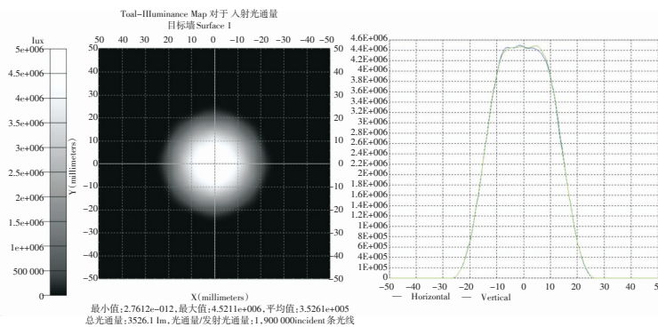
图10 1-8圆形阵列照度分布
