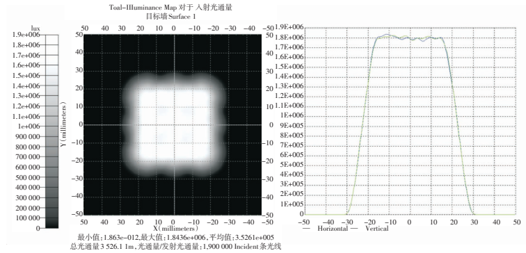
图3 3×3方形阵列照度分布
