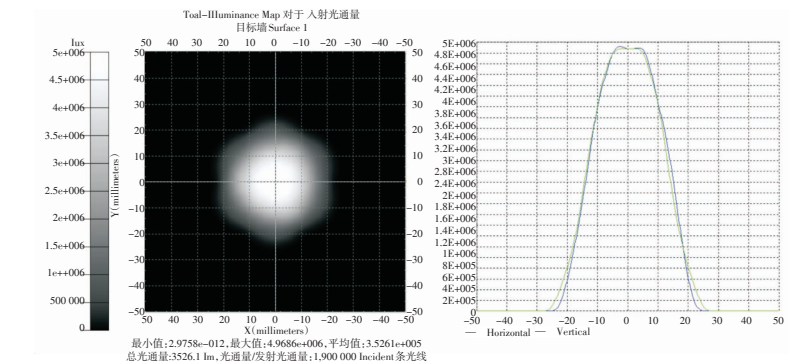
图5 3-6圆形阵列照度分布
