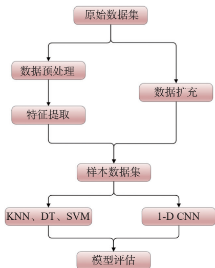
图 1 拉曼光谱分类流程图
