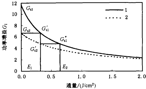
图3 增益通量曲线与小信号增益的关系
