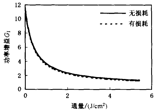
图 1 放大器增益通量曲线
