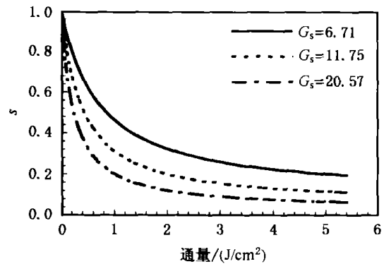
图 2 激光通量对输出波形的影响
