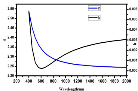
图5 ZnS光学常数拟合结果
