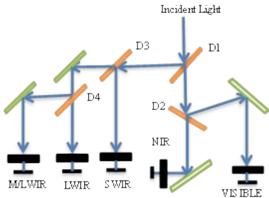
图1 MERSI-III光路排布示意图 Fig. 1 MERSI-III optical layout
