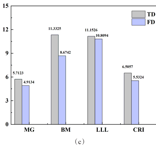
图7 不同孔隙率量化模型的评价比较: (a) R^2 和 R^2_{CV} ; (b) RMSE 和 RMSE_{CV} ; (c) 相对分析误差 RPD Fig. 7 Comparison of the quantitative performances of different porosity models: (a) the values of R^2 and R^2_{CV} ; (b) the values of RMSE and RMSE_{CV} ; (c) the values of RPD
