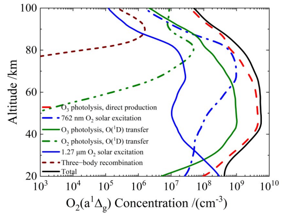
图2 不同物理及化学机制下产生的O 2 (a 1 Δ g )浓度
