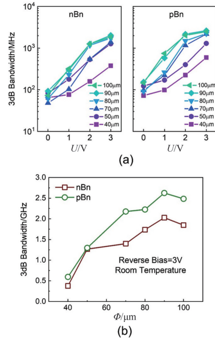
图 6 不同尺寸的 nBn 和 pBn 探测器:(a) -3 dB 截止频率随反向偏压的变化曲线;(b) 在 3 V 反向偏压下的 -3 dB 截止频率随台面直径的变化曲线
