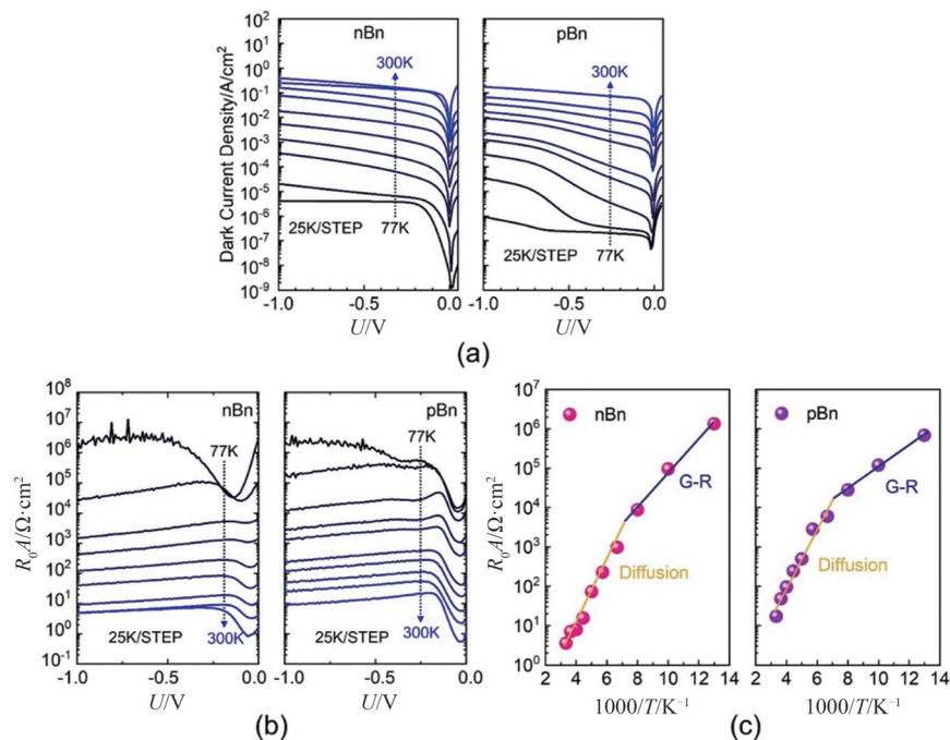
图2 77~300 K温度下直径90 \mu\text{m} 的nBn和pBn探测器单管芯片:(a)暗电流密度-电压曲线;(b)微分电阻和器件面积的乘积 R_0A 随反向偏压的变化曲线;(c) R_0A 随 1000/T 的变化曲线
