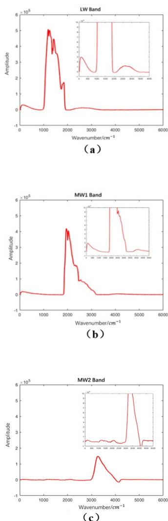
图4 实测光谱数(a)长波,(b)中波1,(c)中波2
