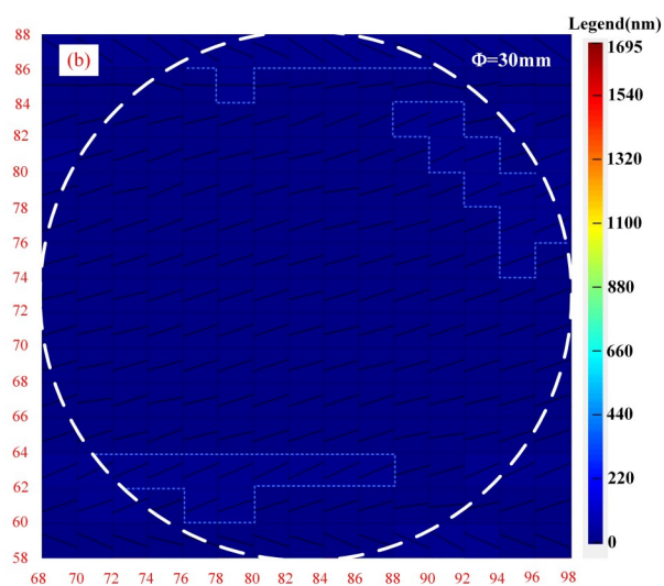
图4 Ge样品的应力双折射延迟量二维分布测试结果(a)Ge样品,(b)应力双折射延迟量分布
