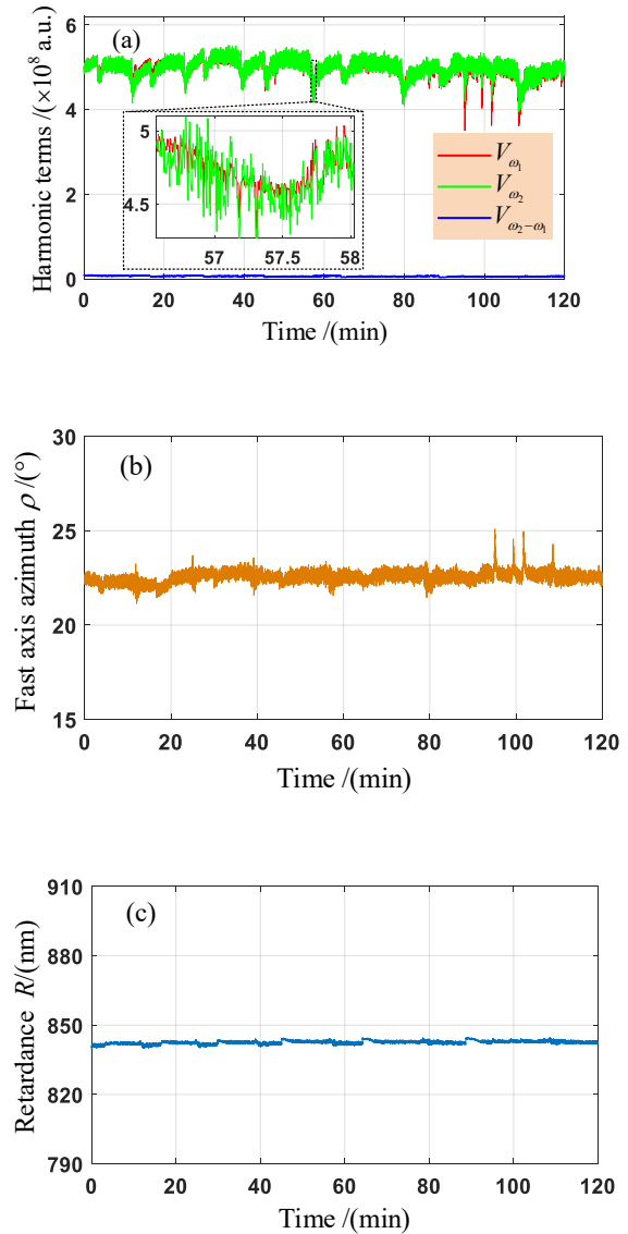
图 3 1/4 波片测试结果 (a) 倍频幅值, (b) 快轴方位角, (c) 延迟量
