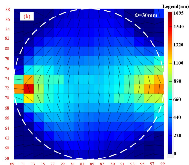
图5 施加力后的Ge样品的应力双折射延迟量二维分布测试结果(a)Ge样品,(b)应力双折射延迟量分布
