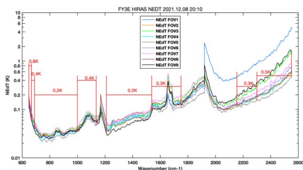
图2 2021年12月8日FY-3E HIRAS-II的NEdT谱分布 Fig. 2 The NEdT distribution of FY-3E HIRAS-II on December 8, 2021
