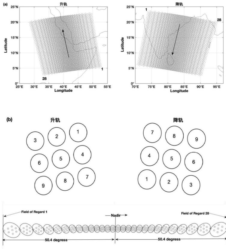
图1 FY-3E/HIRAS-II(a)升降轨每条扫描线以及每个驻留视场的分布(图中箭头为卫星飞行方向), (b)每个FOR中9个FOV的分布
