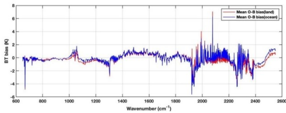
图3 FY-3E/HIRAS-II O-B平均偏差随光谱的分布(红线为陆地,蓝线为海洋)
