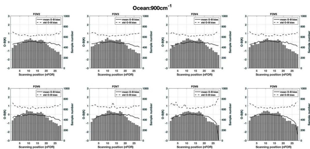
图5 FY-3E/HIRAS-II长波窗区通道 900\text{ cm}^{-1} 各个FOV的O-B平均偏差和偏差标准差随扫描角的分布
