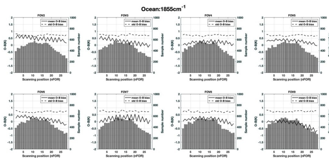
图6 同图5,通道 1855\text{ cm}^{-1}
