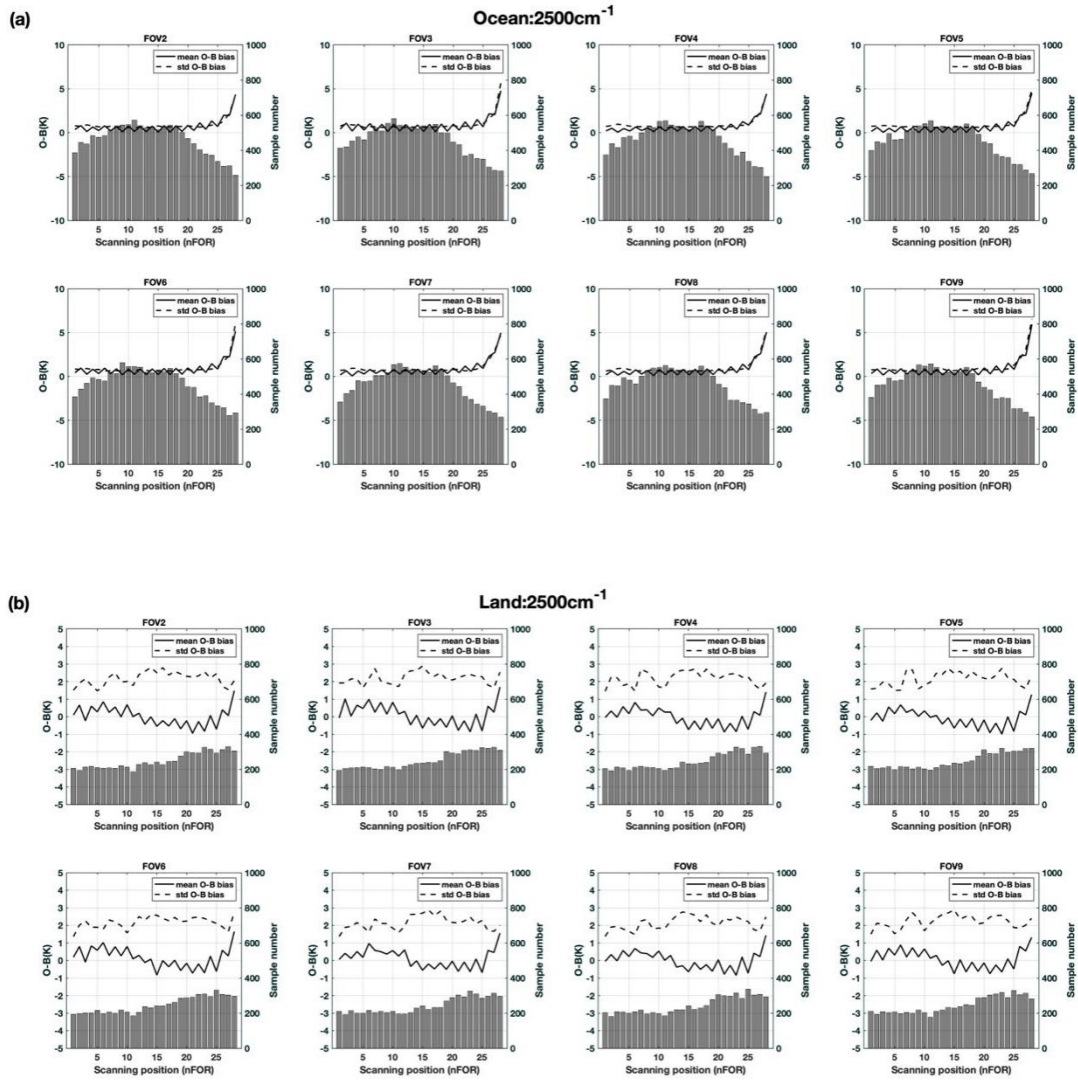
图7 FY-3E/HIRAS-II 短波红外通道 2500\text{ cm}^{-1} 各个 FOV (a)海洋和(b)陆地 O-B 平均偏差和偏差标准差随扫描位置的分布
