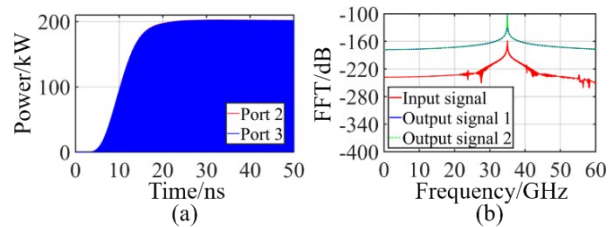
Fig. 13 (a) The output power versus time, (b) the FFT amplitude of the input signal, and output signals from port 2 and port 3 (Output signal 1 and 2 are extracted from port 2 and port 3) 图 13 (a) 输出功率随时间变化图, (b) 输入信号和端口 2、3 的输出信号的快速傅里叶变换幅值 (从端口 2 和端口 3 提取得到输出信号 1 和 2)
