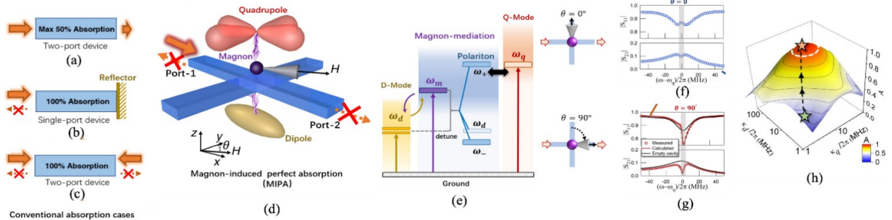
图 7 对称双端口中的电磁吸收限制和单端口系统中的完美吸收的示意图分别显示在 (a) 和 (b)。 (c) 相干完美吸收 (CPA) 策略显示在双端口系统中。 (d) MIPA 系统显示, 通过混合光子-磁子模式之间的干涉实现近乎完美的吸收。能量级示意图见 (e)。在 \theta=0^\circ 和 90^\circ 的反射和传输的平方振幅显示在 (f) 和 (g)。最大吸收的理论函数显示在 (h) 中, 黄色标记表示与非优化设计的绿色标记相比, 修改后的腔体的性能。白色的虚线表示最大吸收率超过 90% [85]
