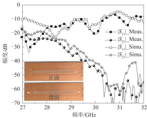
图5 四波束漏波天线实物及仿真和测试 S 参数
