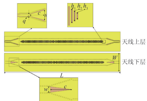
图 4 天线上下层结构图
