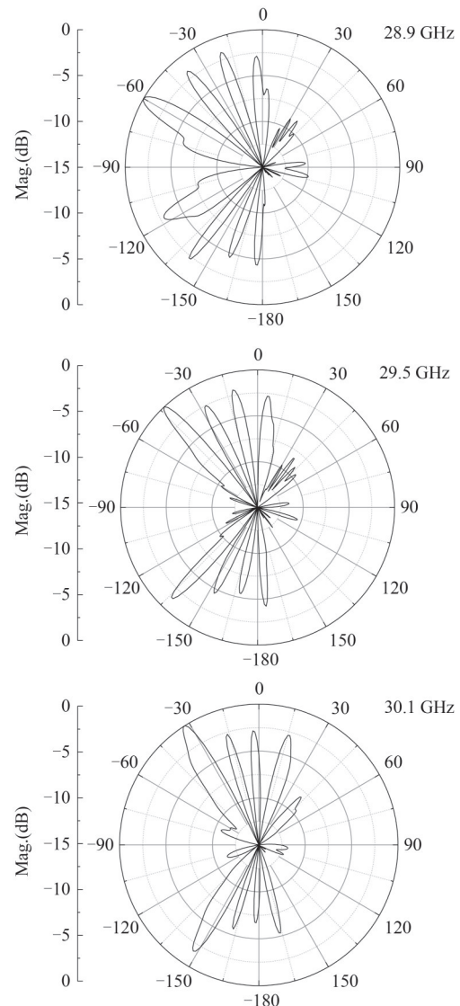
图6 天线在不同频点的归一化远场辐射仿真结果
