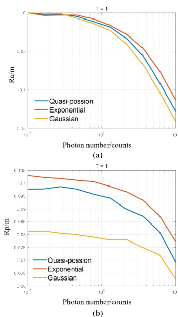
图 12 当阈值 T=1 时,三种脉冲高度分布函数的测距行走误差、测距精确度与入射光子数之间的关系:(a)测距行走误差, (b)测距精确度
