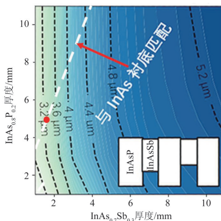
图1 \mathbf{k}\cdot\mathbf{p} 法计算的不同厚度 \text{InAs}_{0.8}\text{P}_{0.2}/\text{InAs}_{0.7}\text{Sb}_{0.3} 超晶格材料截止波长
