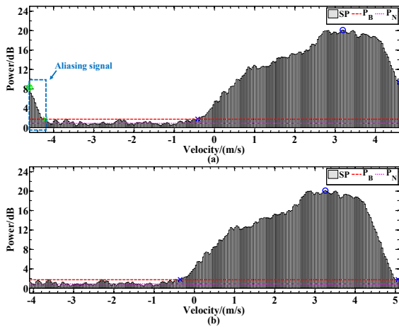
图2 那曲 2015 年 8 月 2 日 23:21 雷达在层积云 3.06 km 处探测的功率谱, (a) 和 (b) 分别为原始谱和纠正后的谱, 图中叉号和圆圈分别代表云雨信号的起终端点和谱峰
