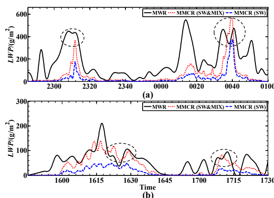
图7 雷达(MMCR)和微波辐射计(MWR)反演的液态水路径 LWP ( g/m^2 )对比,(a)和(b)分别为个例一和个例二
