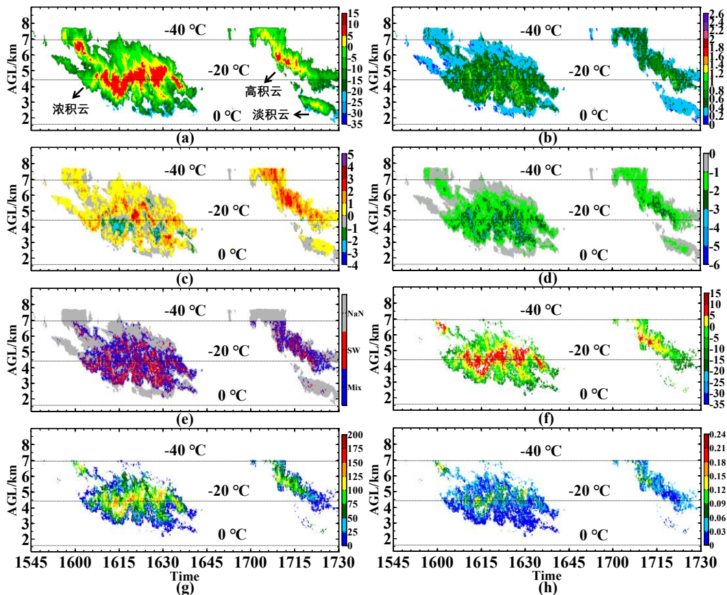
图5 那曲2015年8月25日15:45 - 17:30浓积云、高积云和淡积云(个例二)的雷达探测和反演结果,各子图含义同图4
