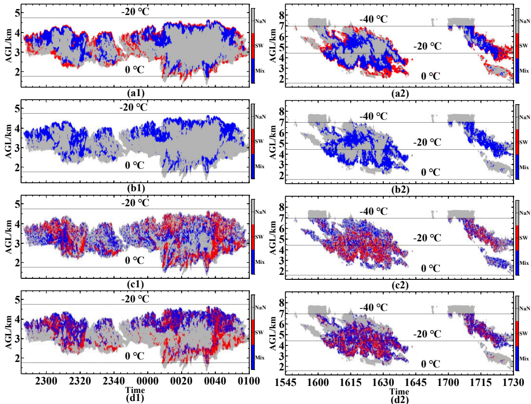
图 8 两次个例使用不同方法反演的过冷水空间分布结果,(a1, a2) 模糊逻辑算法 FHC,(b1, b2) 阈值法 Threshold,(c1, c2) K-均值聚类算法 K-means,(d1, d2) 本文方法 Our Method
