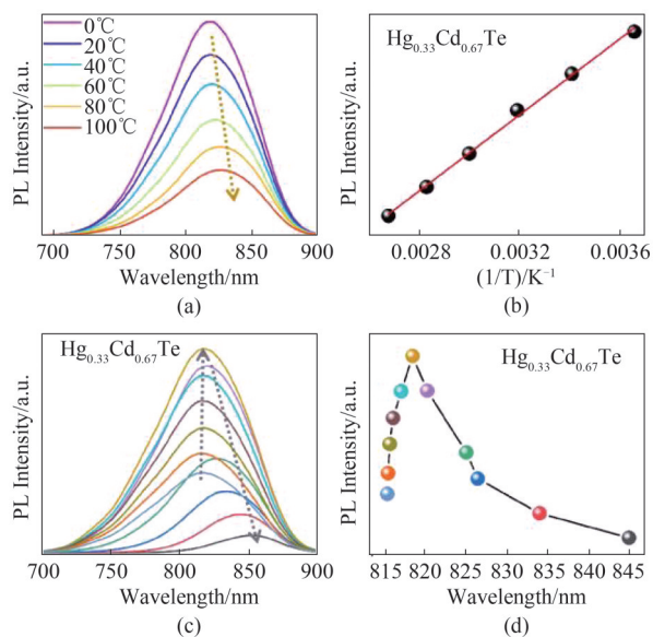
图5 (a) \text{Hg}_{0.33}\text{Cd}_{0.67}\text{Te} 量子点在0-100°C下的变温荧光光谱图,(b)荧光强度和温度之间变化关系,(c) \text{Hg}_{0.33}\text{Cd}_{0.67}\text{Te} 量子点随浓度变化的荧光发射图谱,(d)相应荧光发射强度与峰位变化情况
