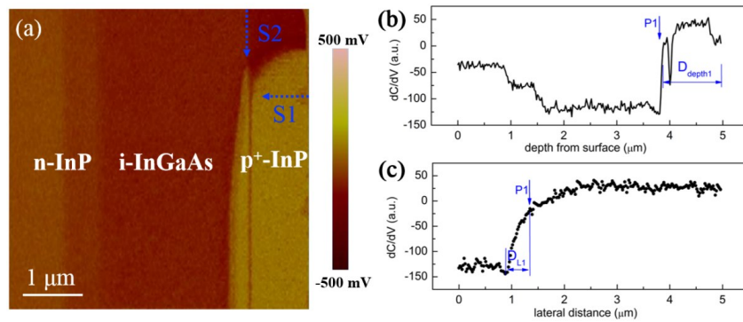
图3 (a) InGaAs/InP P-i-N探测器器件结构的SCM图, (b) 沿S1方向的SCM曲线, (c) 沿S2方向的SCM曲线
