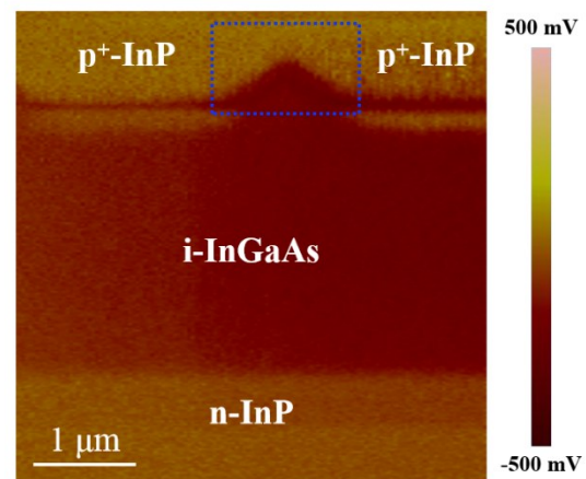
图4 InGaAs/InP P-i-N探测器中因侧向扩散引起相连缺陷元的SCM图
