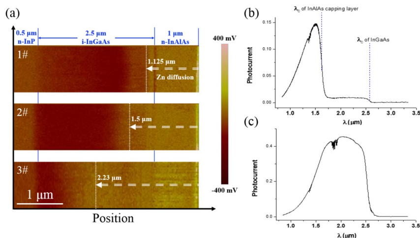
图2 (a) 三种不同扩散深度的 InGaAs/InAlAs 探测器 SCM 图, (b) 杂质扩散在 InAlAs 帽层以及进入 InGaAs 吸收层两种情况下的器件光电流响应
