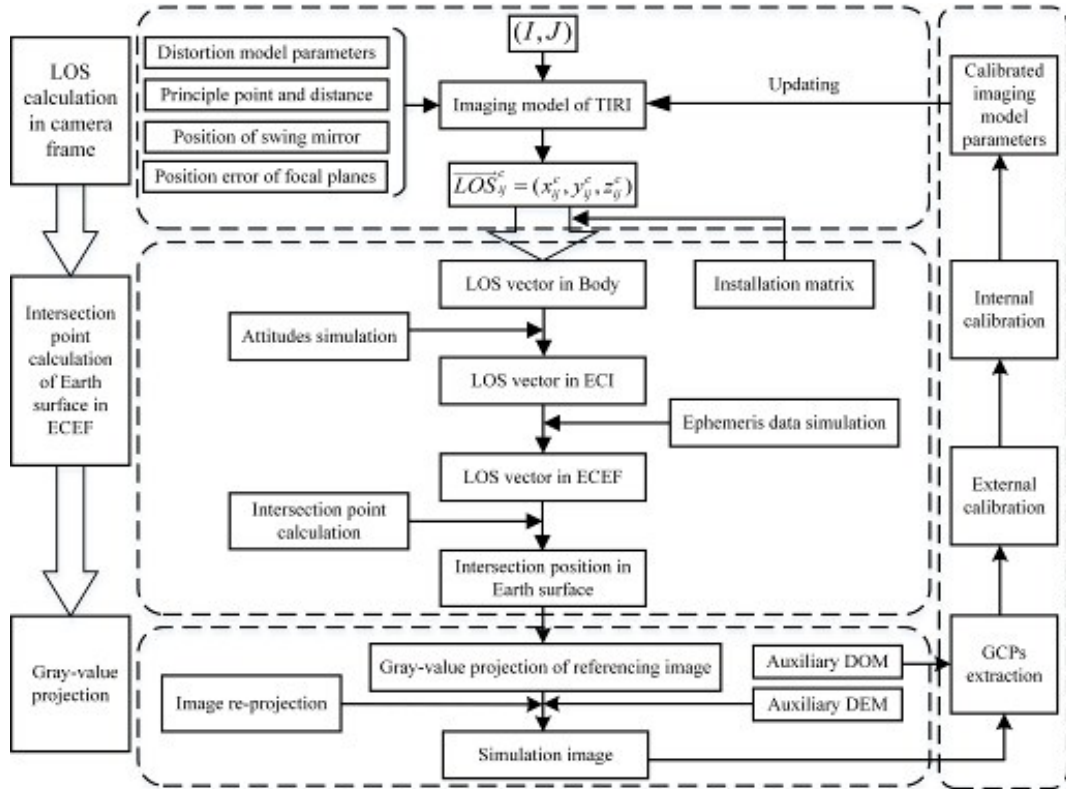
图2 热像仪在轨几何成像仿真流程
