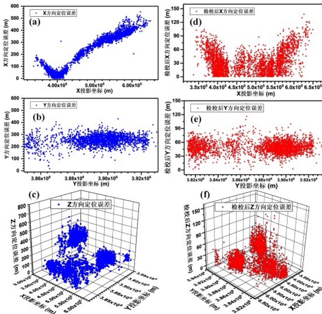
图5 校正前后仿真影像几何定位误差分布对比:(a)校正前X方向定位误差,(b)校正前Y方向定位误差,(c)校正前Z方向定位误差,(d)校正后X方向定位误差,(e)校正后Y方向定位误差,(f)校正后Z方向定位误差
