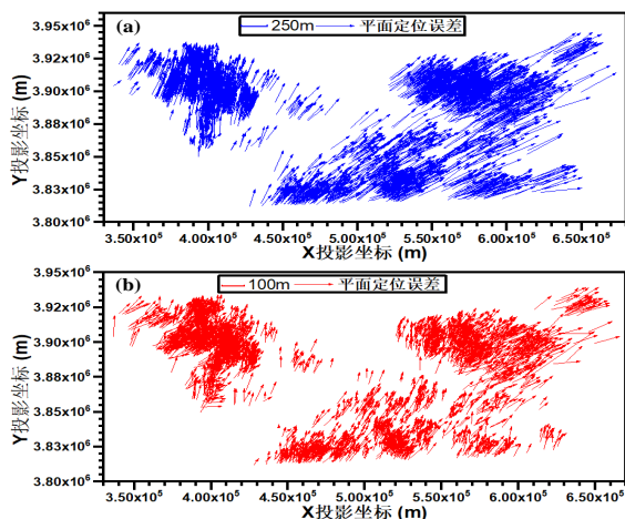
图6 校正前后仿真影像平面几何定位误差分布对比:(a)校正前平面定位误差,(b)校正后平面定位误差
