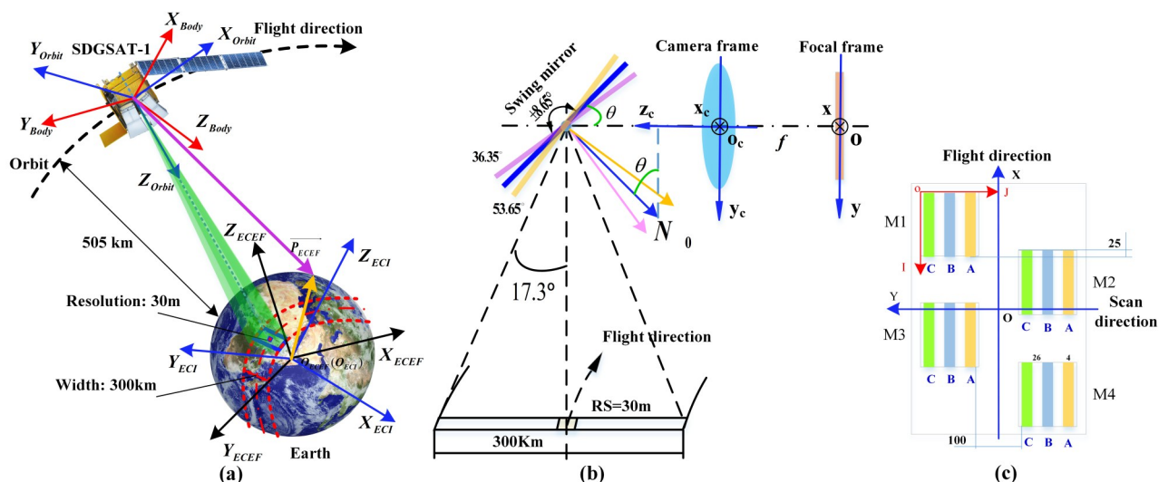
图 1 热像仪在轨成像、光路及探测器排列示意图(a)在轨成像示意图,(b)光路示意图,(c)探测器拼接示意图
