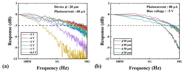
图6 (a) 室温下5级带间级联探测器在不同偏压下频率响应曲线,(b) -5 V偏压不同面积器件频率响应曲线 [25]
