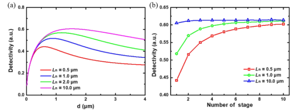
图2 (a) 单吸收区结构量子效率与吸收区厚度关系,(b) 光电流匹配结构在不同的扩散长度和级数下能达到的最大探测率
