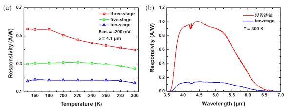
图 4 (a) 3 级、5 级和 10 级带间级联探测器响应率随温度变化关系, (b) 制备了浸没透镜和减反膜后 10 级带间级联探测器响应率
