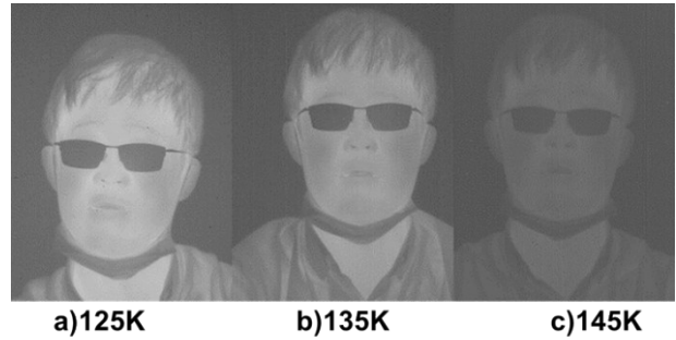
图 5 带间级联中波红外焦平面变温成像演示,工作温度分别为 (a) 125 K, (b) 135 K, (c) 145 K
