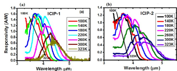
图3 (a) 1级和(b) 2级带间级联探测器的变温响应光谱 [23]
