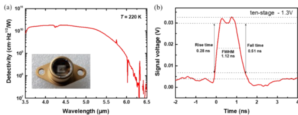
图7 (a) 10级带间级联探测器探测率曲线,(b) -1.3 V偏压下器件响应时间曲线,插图是热电制冷封装10级带间级联探测器示意图
