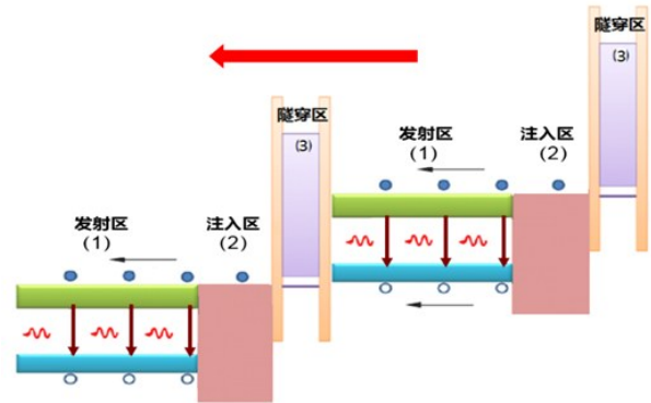
图8 带间级联LED能带结构示意图
