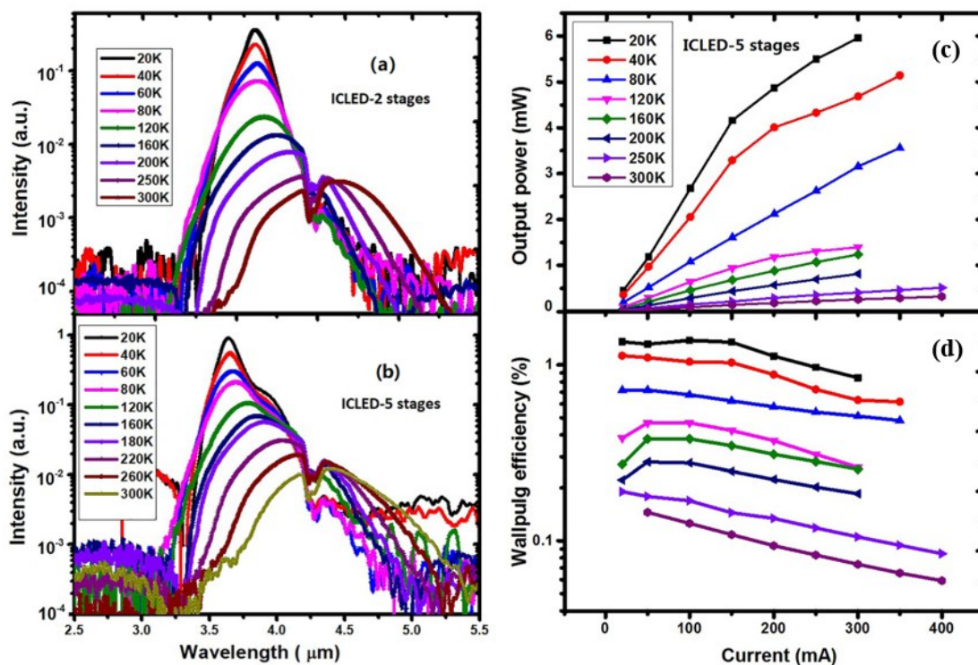
图9 (a) 2级带间级联LED发光光谱, (b) 5级带间级联LED发光光谱, (c) 5级带间级联LED发光功率, (d) 5级带间级联LED电光转化效率(面积 400 \times 400 \mu\text{m}^2 ) [26]
