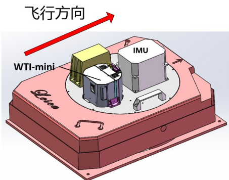
图 17 SIRI-4 集成在 PAV-80 平台 Fig. 17 SIRI-4 is integrated on the PAV-80 platform
