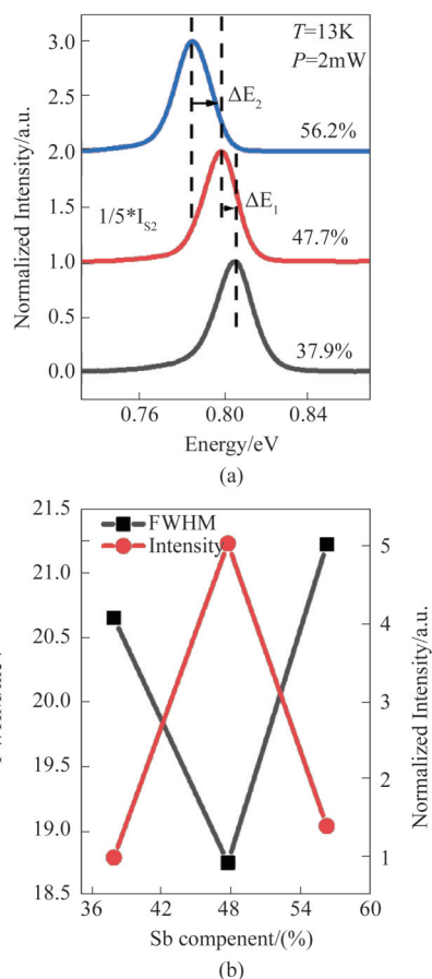
图2 (a) 三块样品S1(Sb=37.9%)、S2(Sb=47.7%)和S3(Sb=56.2%)在13 K下,功率为2 mW的荧光发光光谱, (b) PL光谱的半峰宽和强度的组分依赖关系趋势图
