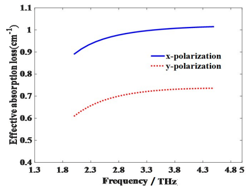
图 7 当 r=2 \mu\text{m} , L=14.5 \mu\text{m} , d=29 \mu\text{m} , R=49 \mu\text{m} , \Lambda=100 \mu\text{m} 时, 2~4.5 THz 频率范围内光纤的有效吸收损耗曲线
