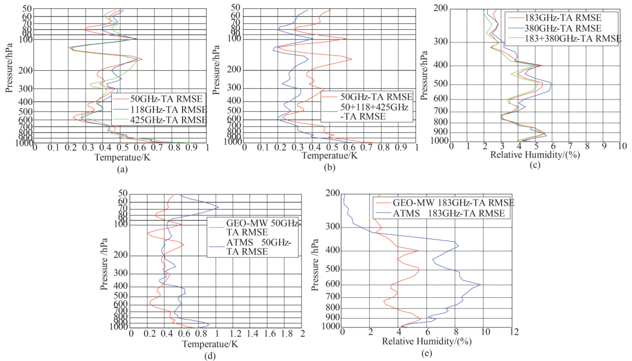
图7 不同频段亮温 T_A 反演大气温湿廓线的 RMSE 对比(a)50 GHz、118 GHz、425 GHz 反演的温度廓线 RMSE, (b)50 GHz 和三个频段组合反演的温度廓线 RMSE, (c)183 GHz、380 GHz 和两个频段组合反演的湿度廓线 RMSE, (d)50 GHz 静止轨道和 ATMS 亮温反演的温度廓线 RMSE, (e)183 GHz 静止轨道和 ATMS 亮温反演的湿度廓线 RMSE
