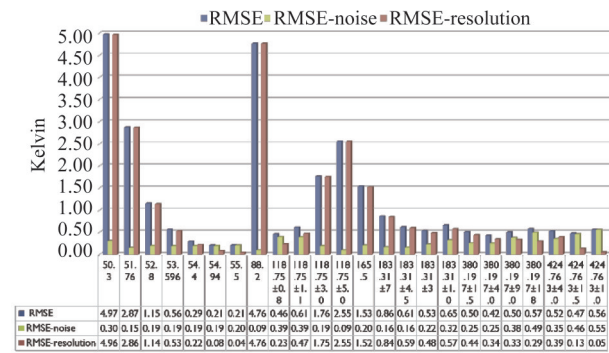
图6 飓风桑迪静止轨道观测亮温误差
