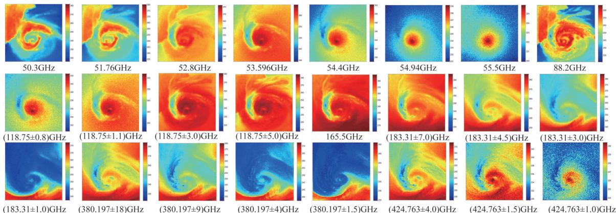
图 5 飓风桑迪静止轨道模拟观测亮温图像
