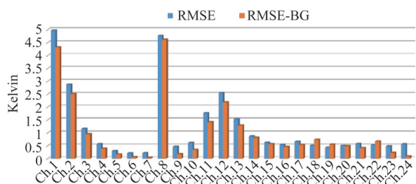
图10 观测亮温 T_A 和BG重建亮温 T_{A\_BG} 的RMSE对比
