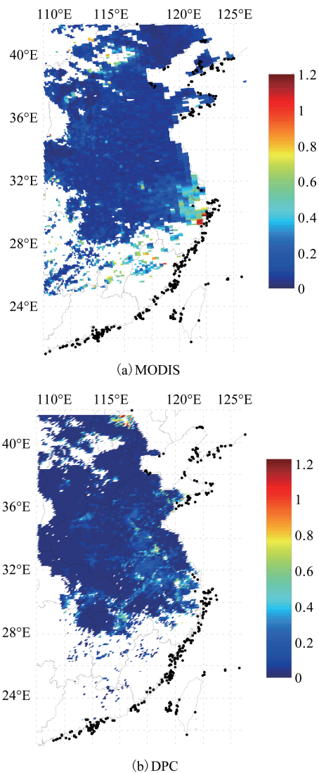
图1 2018年9月4号DPC和MODIS气溶胶产品对比结果 Fig.1 Comparison of DPC and MODIS retrieved AOD on September 4, 2018
