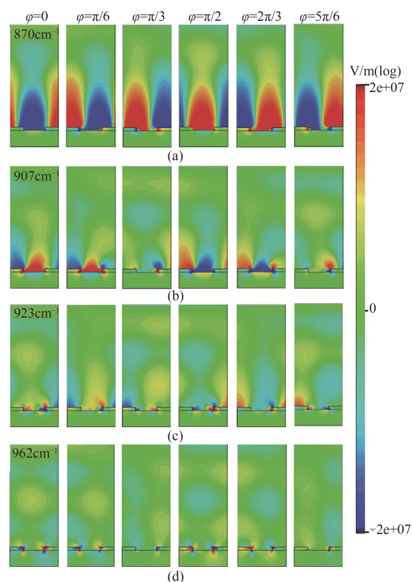
图2 四种模式电场分布演化图
