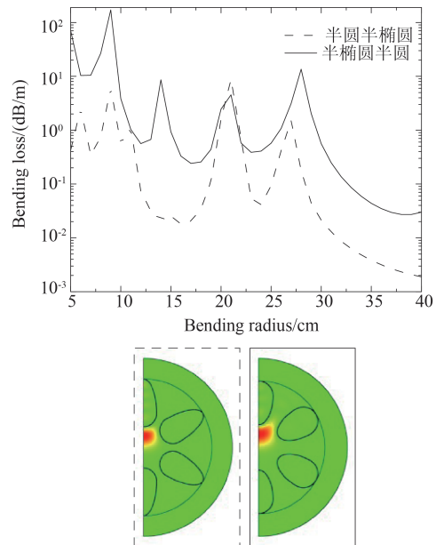
图 8 两种改进结构的弯曲损耗与弯曲半径的函数关系(左);两种结构的模场图(右)
