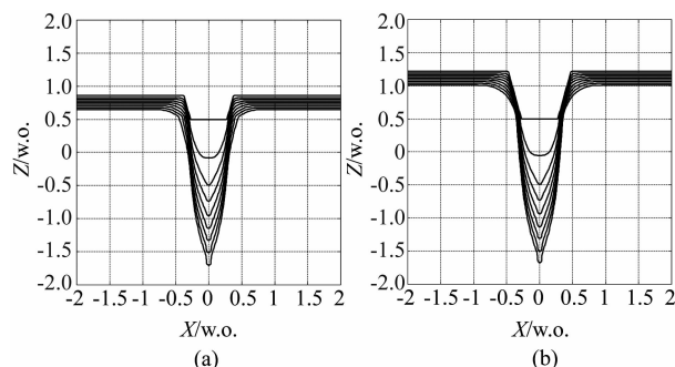
图10 名义沟槽宽度为 4 \mu\text{m} ,刻蚀时间为4.5小时的碲镉汞轮廓演变的模拟结果,掩膜厚度:(a) 3.6 \mu\text{m} , (b) 7.2 \mu\text{m} . 轮廓中 Z > 0.5 的部分为掩膜, Z \leq 0.5 的部分为碲镉汞
