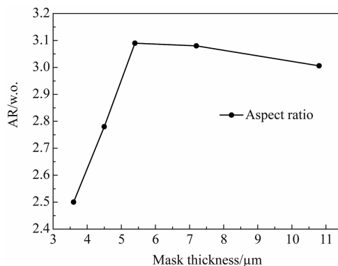
图11 碲镉汞的深宽比随掩膜厚度变化的关系,名义沟槽宽度为 4 \mu\text{m} ,刻蚀时间为4.5小时
