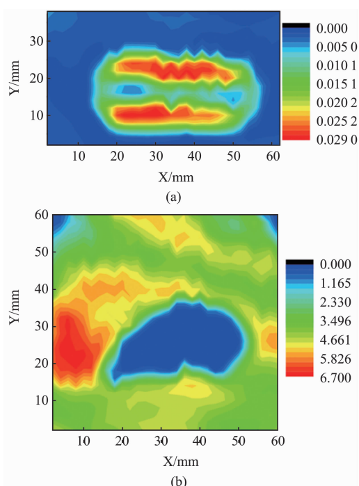
图 8 太赫兹波反射成像效果图: (a) 刀片成像, (b) 矿石成像
