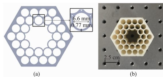
图2 (a) 波导横截面设计图,(b) 波导实物图 Fig. 2 (a) Cross section of waveguide design,(b) Photograph of fabrication waveguide
