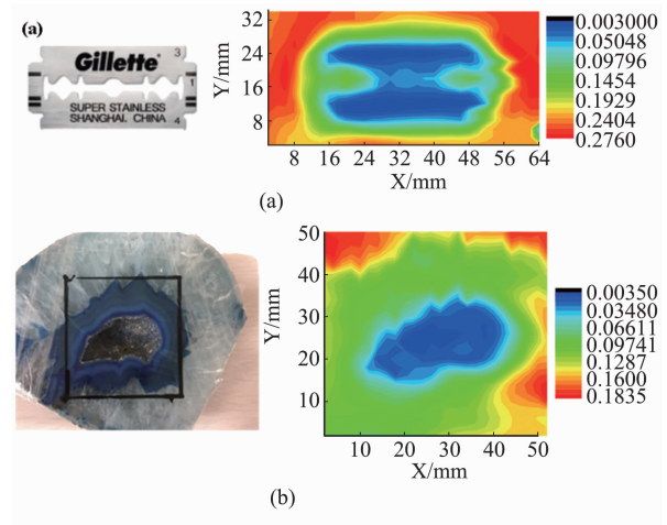
图 6 太赫兹波透射成像效果图: (a) 刀片成像, (b) 矿石成像 Fig. 6 Terahertz wave transmission imaging: (a) Blade imaging, (b) Ore imaging
