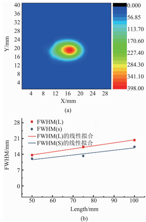
图 5 波导末端发散角测量: (a) 距离波导末端 5 cm 位置处的太赫兹场分布, (b) 发散角测量结果 Fig. 5 The measurement of divergence angle at the waveguide end; (a) Terahertz spot distribution at 5 cm, (b) Divergence angle measurement result
