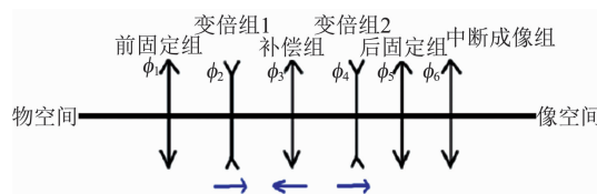
图 1 新型变焦结构型式 Fig. 1 New Zoom Model Structure
