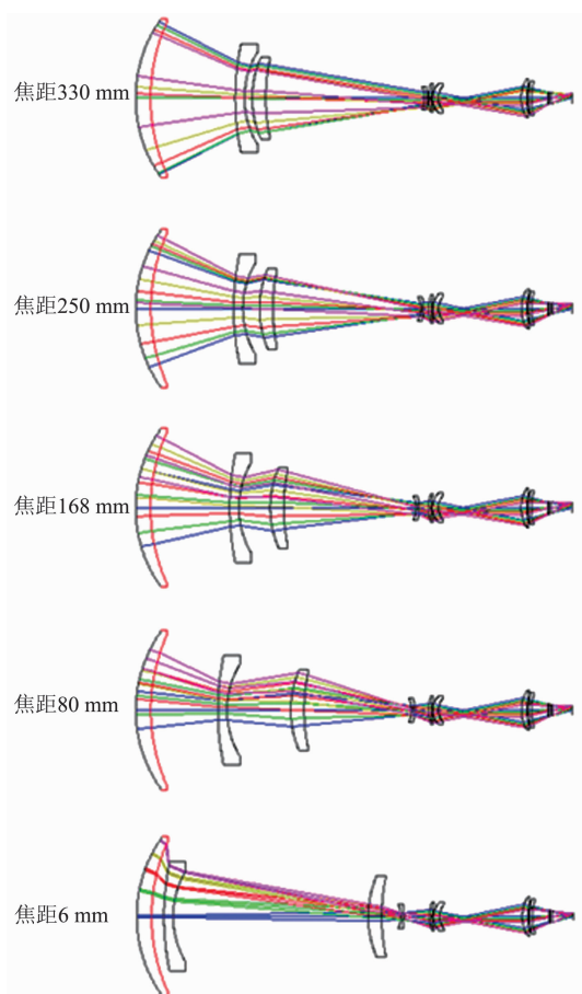
图 2 光学系统光路图
