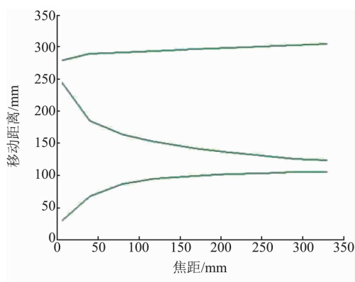
图4 系统变焦曲线图
