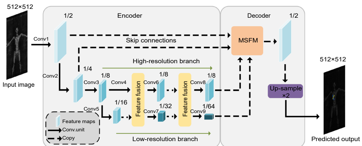
图 1 DBMFnet 网络结构图
