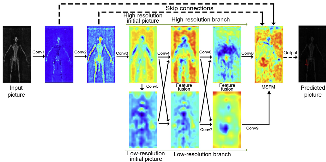
图 5 DBMFnet 热力图
