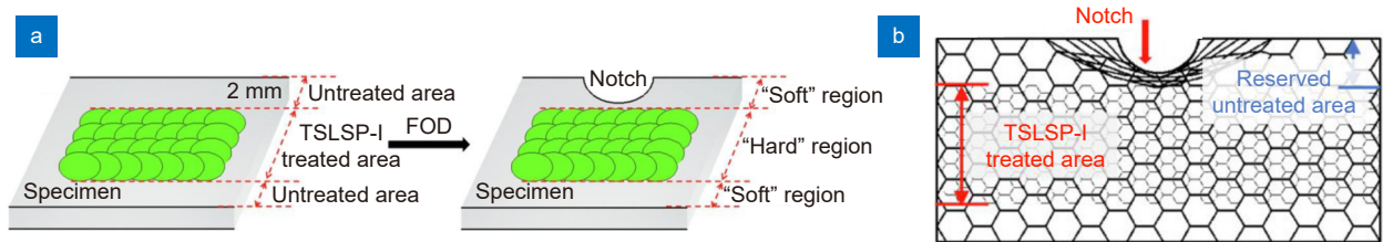
图 18 激光冲击强化产生的软硬交替吸能结构和晶粒分布细化。 [48] (a) 软硬交替吸能结构; (b) 晶粒分布细化 [48]
