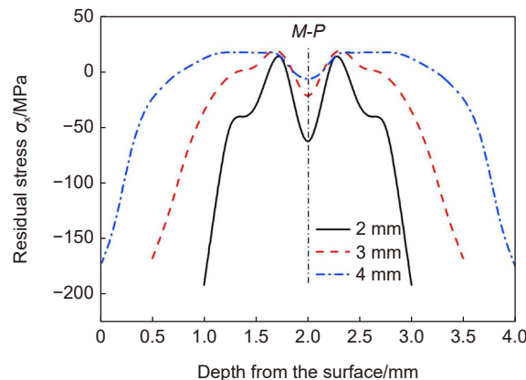
图 20 厚度方向的残余应力随板材厚度的变化 [52]
