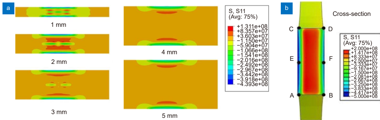
图 8 双面激光冲击强化后的残余应力场。(a) 板材厚度对双面同步激光冲击强化残余应力场影响 [27] ; (b) 双面异步激光冲击强化残余应力场 [34]
